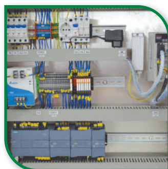
електрошкаф
